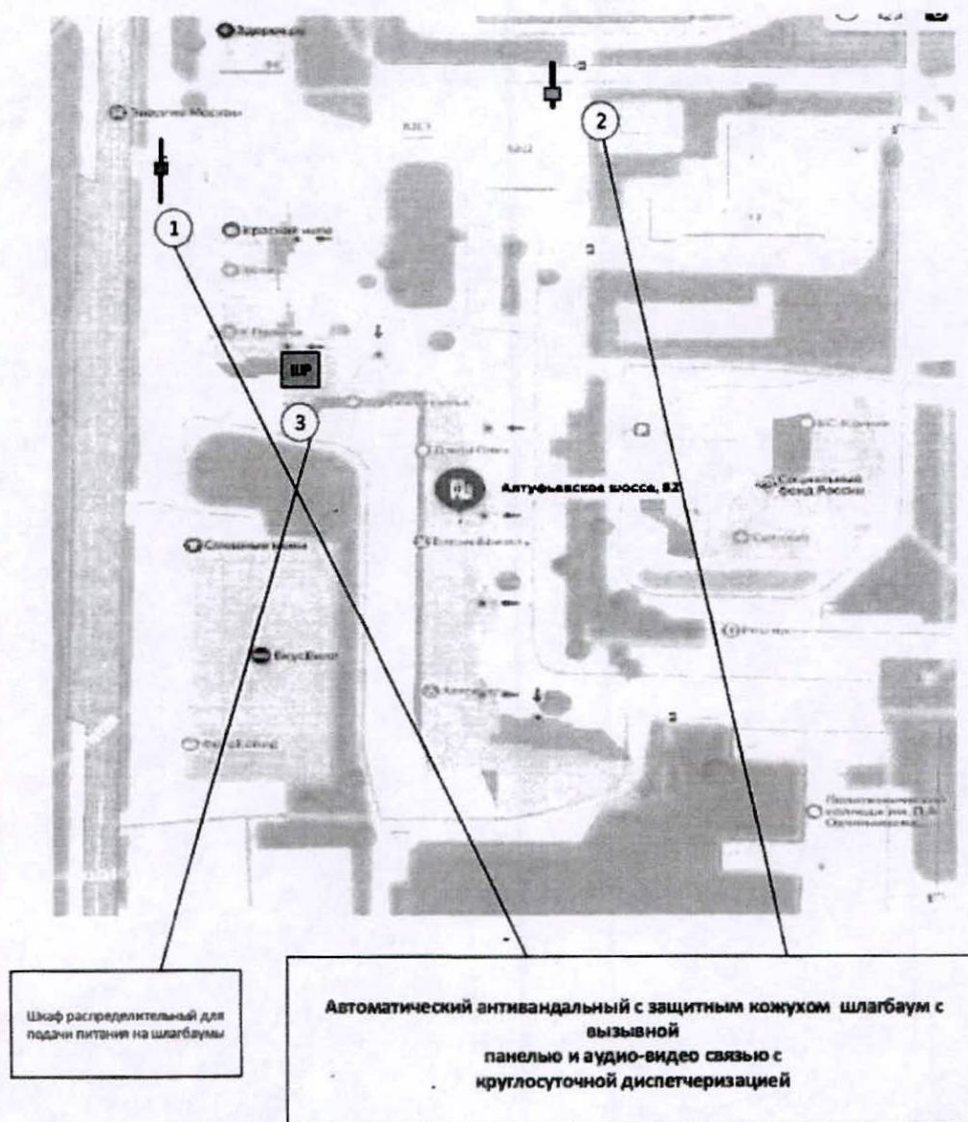
Рис. 1 Схема размещения ограждающих устройств
